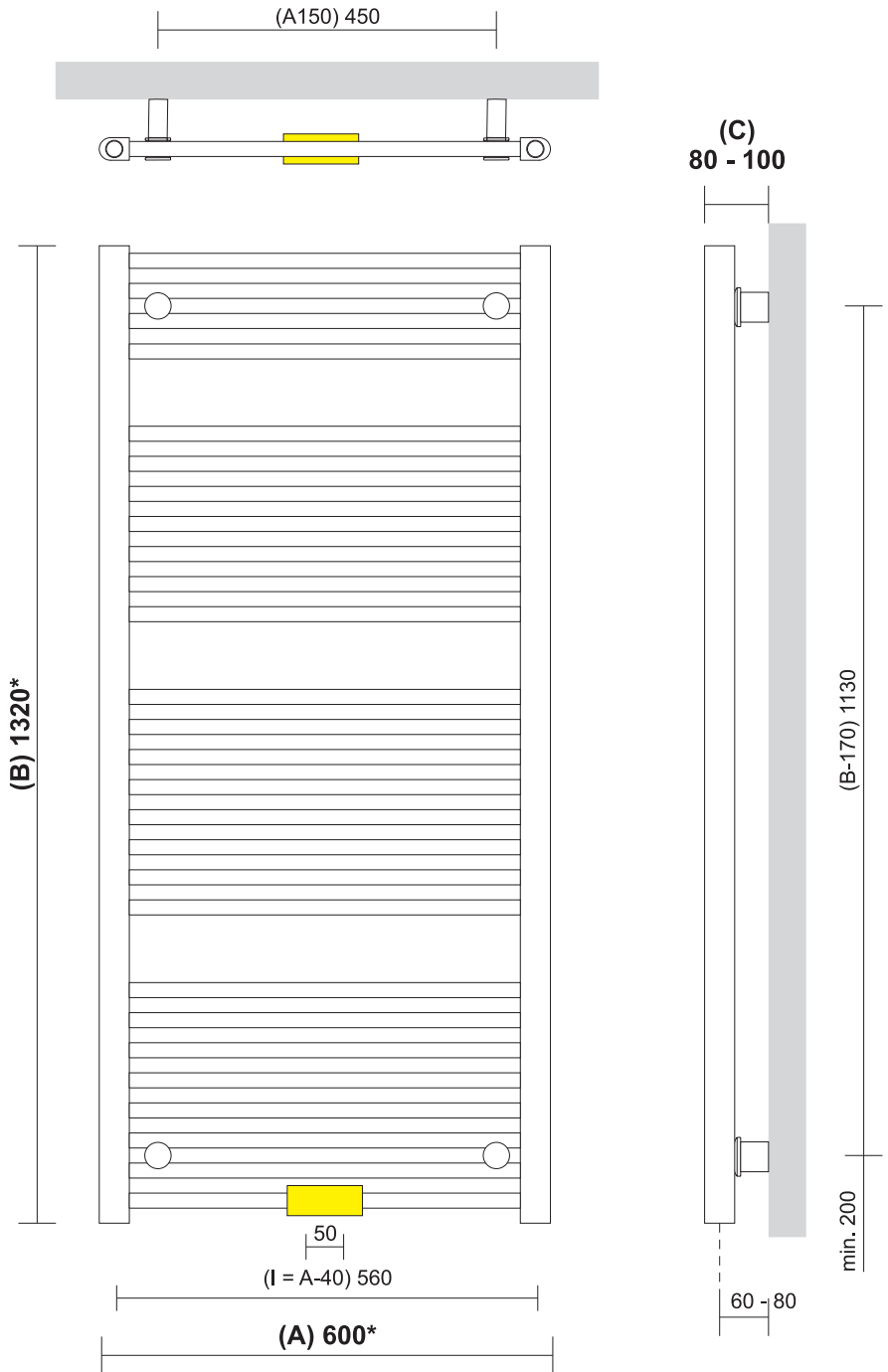
Bild: Laurens Centrix LX 600/1300, 600x1300x80, inkl. Mittelanschluss (Aufpreis) 50mm, M 1:10
